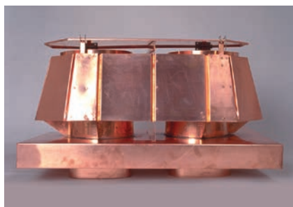
Tipo Standard a 2 canali con copertura
