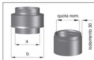
Tipo 1 Anello di dilatazione con risvolto isolamento 30 mm
