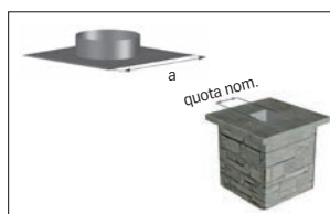
Tipo 2 – sporto quadrato senza raccordo
