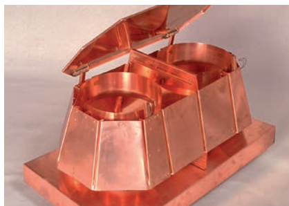
La lamiera di separazione tra i canali del camino impedisce che il fumo possa passare da un camino all'altro.
