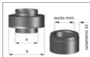
Tipo 1 Anello di dilatazione con risvolto isolamento 50 mm
