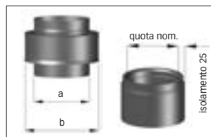
Tipo 1 Anello di dilatazione con risvolto isolamento 25 mm
