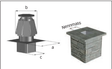
solin carré avec piquage carré
