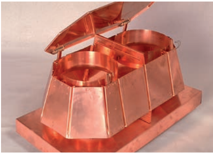
Une tôle de séparation placée entre les conduits empêche que la fumée s'échappant d'une cheminée puisse pénétrer dans une autre.
