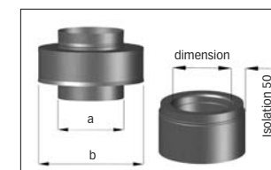
Type 1 anneau de dilation isolation 50 mm
