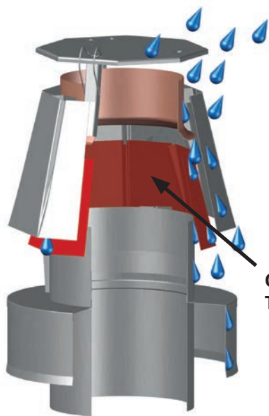
Gaine intérieure Type Régulateur
