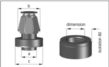
anneau de dilation isolation 80 mm
