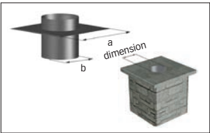
Type 3 – solin carré avec piquage rond
