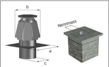
solin carré avec piquage rond
