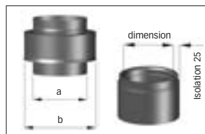
Type 1 anneau de dilation isolation 25 mm
