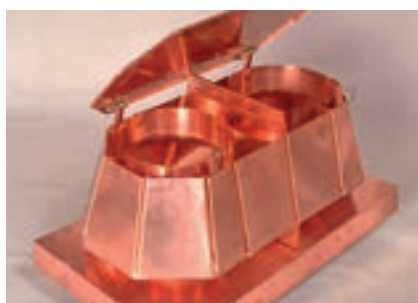
Une tôle de séparation placée entre les conduits empêche que la fumée s'échappant d'une cheminée puisse pénétrer dans une autre.
